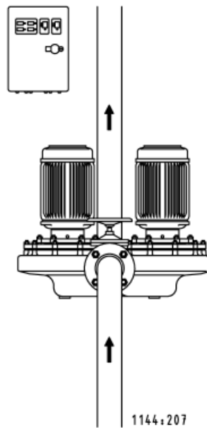
Крепление Trialine Z типоразмеров ...-160/... и ...-250/... с 3 опорными лапами (см. Принадлежности)
