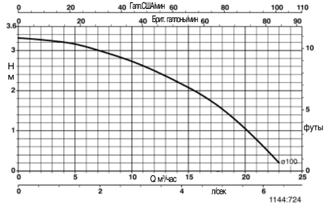
Trialine Z 50-125/024
