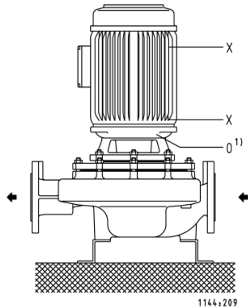
Вертикальный монтаж с тремя опорными лапами
