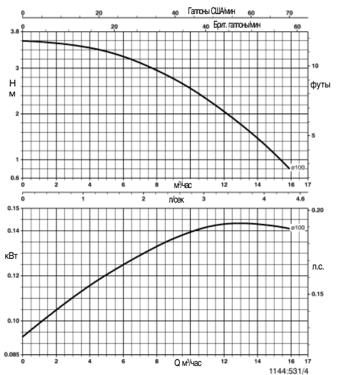
Trialine Z 50-125/024
